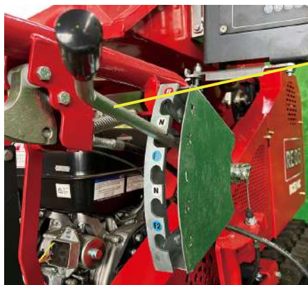
シフトレバー
