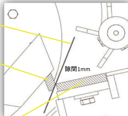
隙間ゲージプレート
