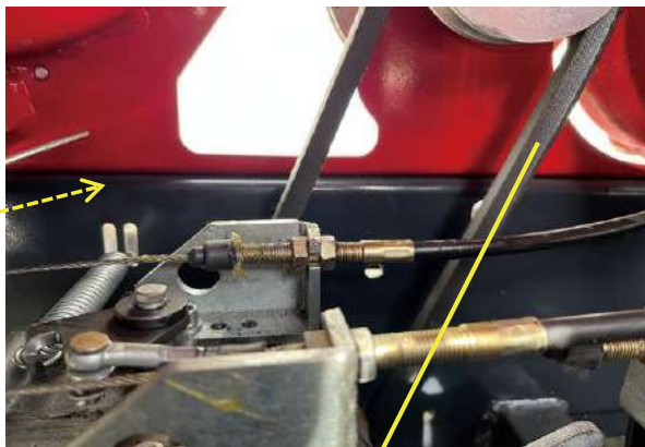
走行ベルト②
