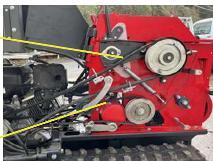
(4) ローターベルト
