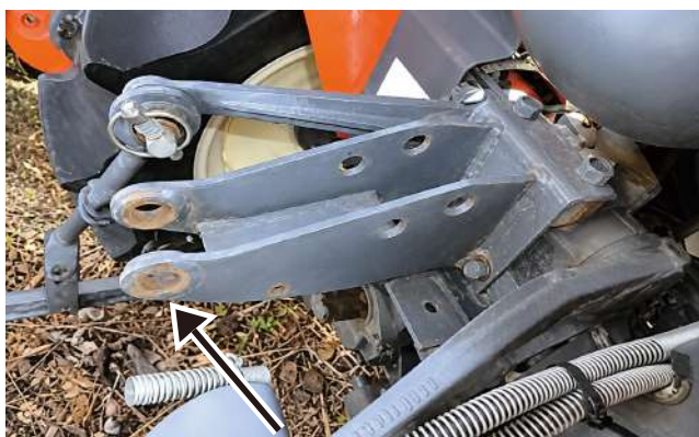
【取付穴の位置】
